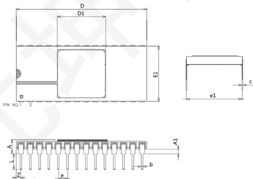
图3-2 YK6664RH (DIP28) 封装外形尺寸示意图
