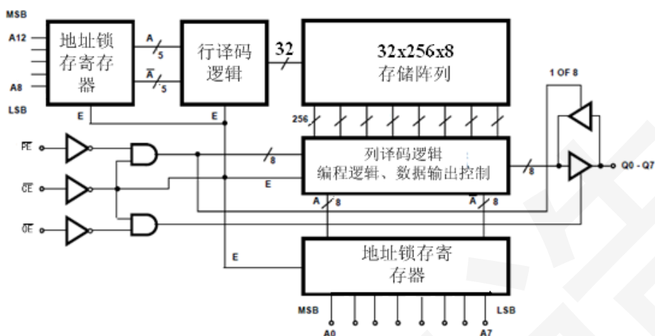
图 4-1 YK6664RH 功能框图
