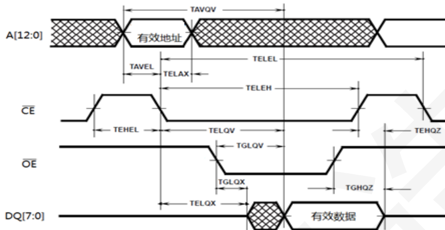
图 5-1 交流参数测试示意图
