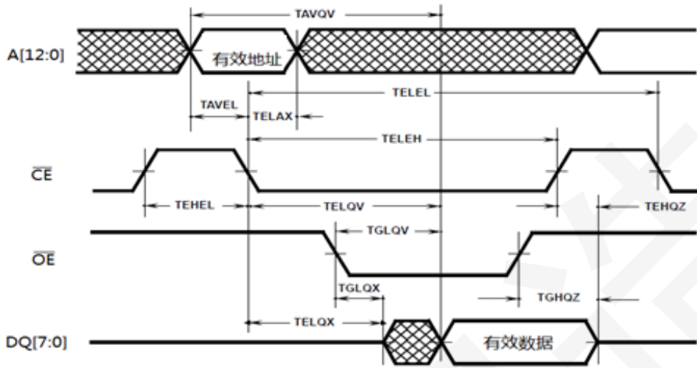
图 4-4 读操作方式 3：输出使能控制读取
