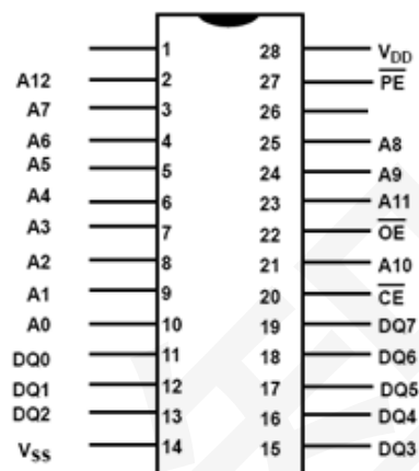
图3-1 YK6664RH引脚排列顺序
