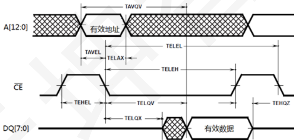
图 4-3 读操作方式 2：片选控制读取
